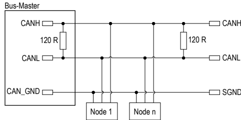
Abb. 4: Terminierung CAN
