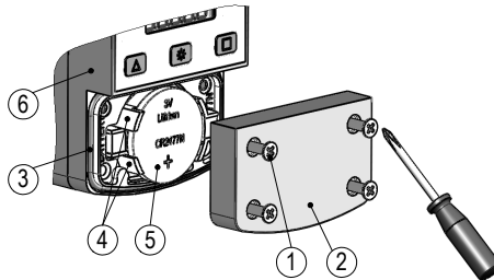
Abb. 9: Batteriewechsel
