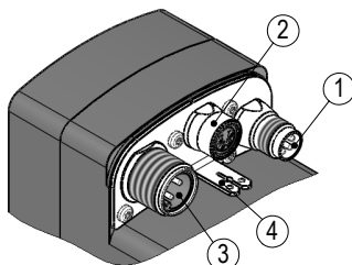
Abb. 6: Anschlussbelegung
