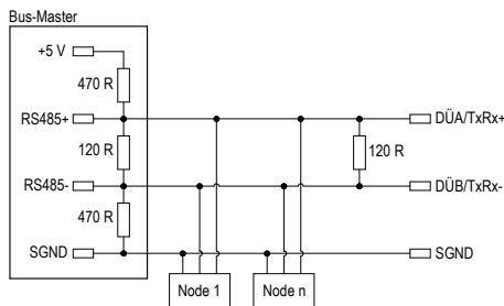
Abb. 5: Terminierung und Pegelfestlegung RS485
