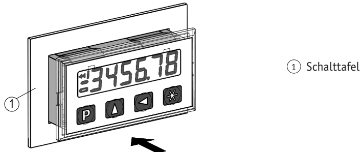
Abb. 2: Montage
