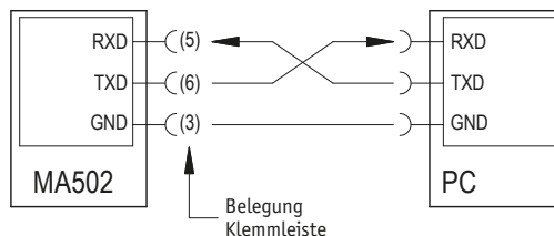
Abb. 4: Anschlusschema Schnittstellenoption RS232
