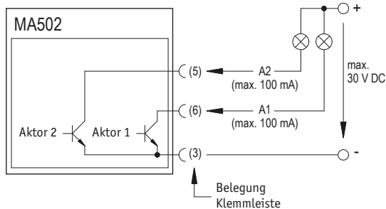
Abb. 6: Anschlusschema Option Schaltausgänge
