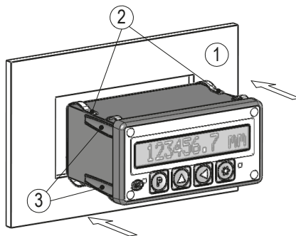
Abb. 1: Einbau
