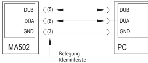
Abb. 5: Anschlusschema Schnittstellenoption RS485
