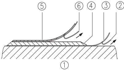
Abb. 1: Montage Magnetband
